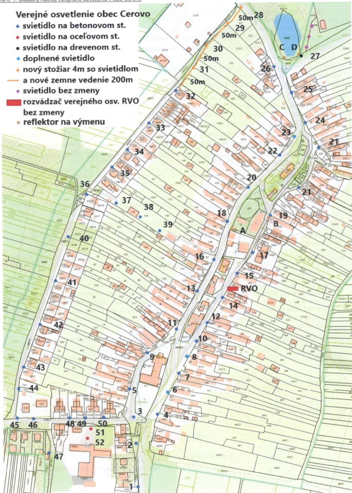
Príloha č. 1: Situačný náčres verejného osvetlenia v obci Cerovo
